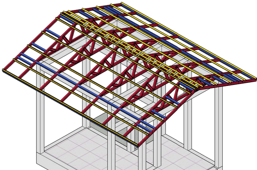
1 STR ISOMETRIK PAS. BAJA RINGAN NS
