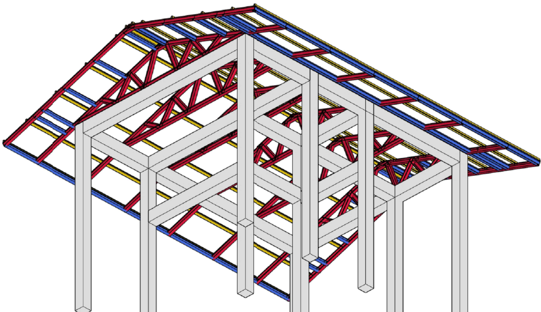
1 STR ISOMETRIK PAS. BAJA RINGAN NS
