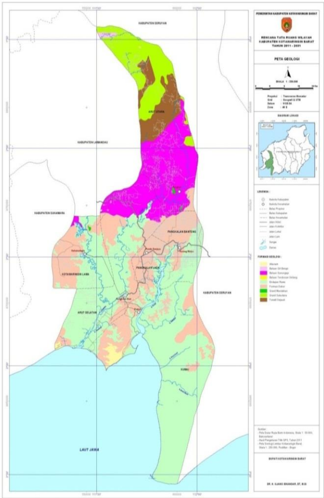
Gambar 3.1 Peta Geologi Wilayah Kabupaten Kotawaringin Barat
