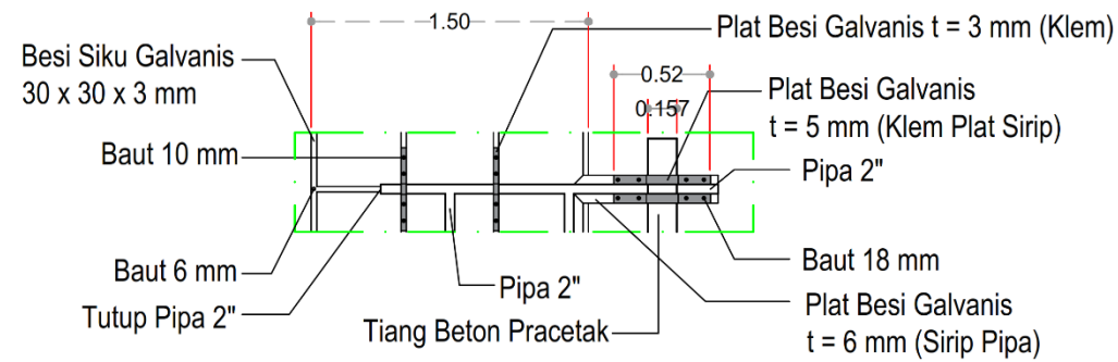
Tampak Belakang Detail Rambu Uk. 150 x 200 cm (Tiang F) Skala 1 : 30
