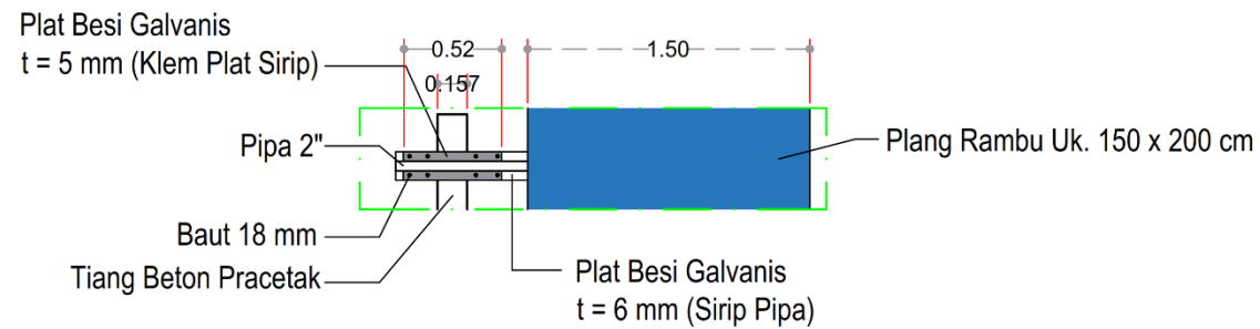
Tampak Depan Detail Rambu Uk. 150 x 200 cm (Tiang F) Skala 1 : 30
