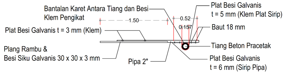
Tampak Atas Detail Rambu Uk. 150 x 200 cm (Tiang F) Skala 1 : 30
