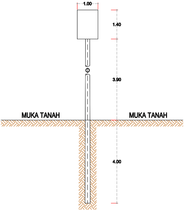
TAMPAK DEPAN Skala 1 : 100
