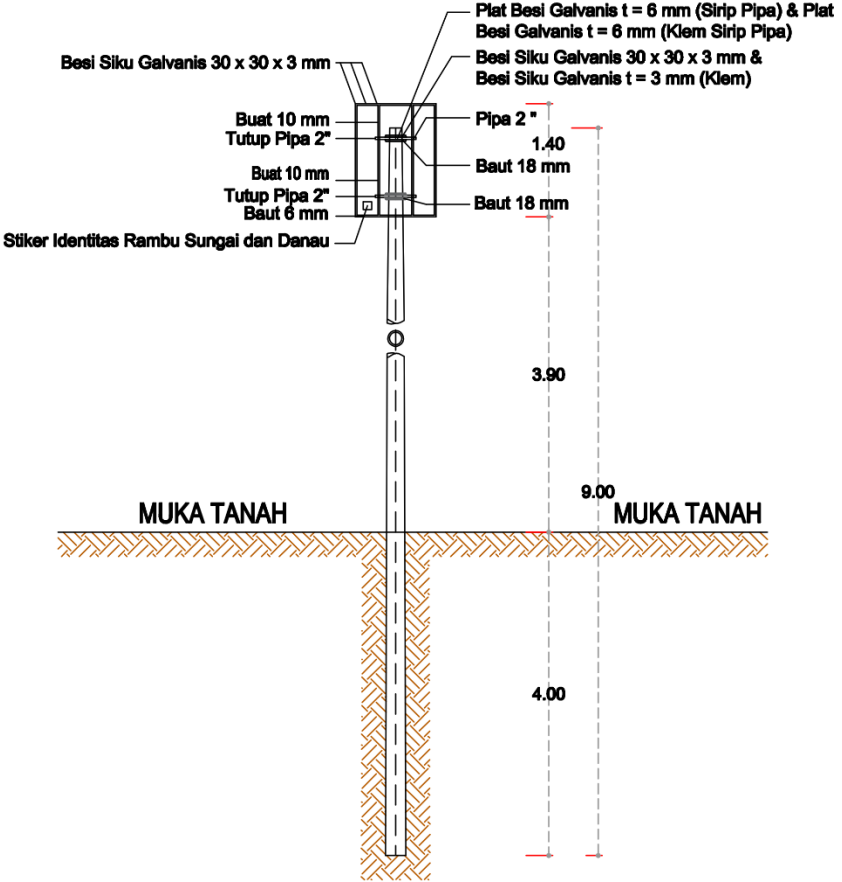
TAMPAK BELAKANG Skala 1 : 100
