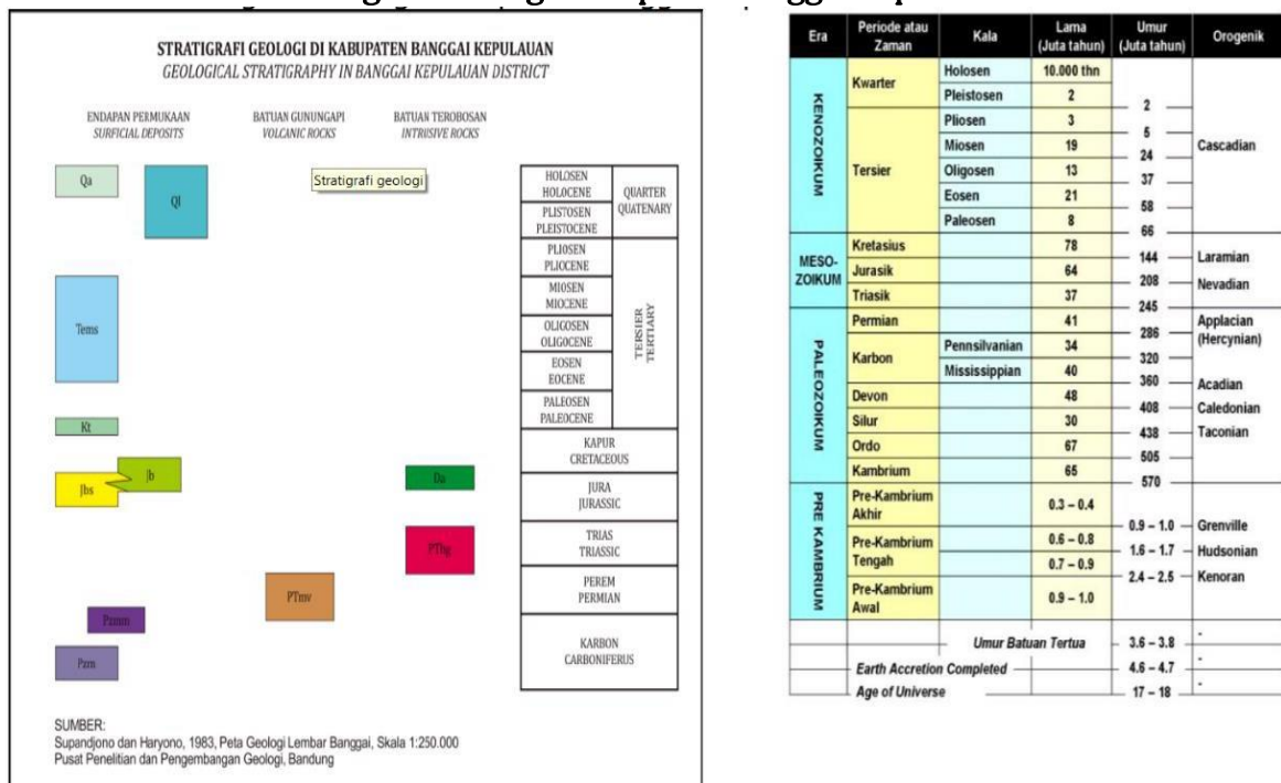
Gambar 2.4 Stratigrafi Geologi Kabupaten Banggai Kepulauan
